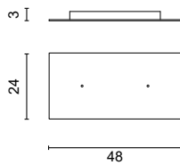
Deckenrosette mit Konverter - 2 Spirits IN 50/60Hz 220-240V
