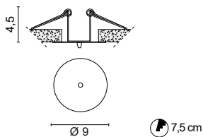
Deckenrosette aus Gipskarton mit Kon- verter 1 Spirits IN 50/60Hz 220-240V
