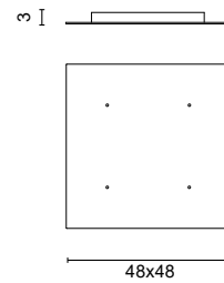
Deckenrosette mit Konverter - 4 Spirits IN 50/60Hz 220-240V
