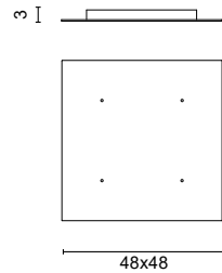
Deckenrosette für 4 Unidea IN 50/60Hz 220-240V
